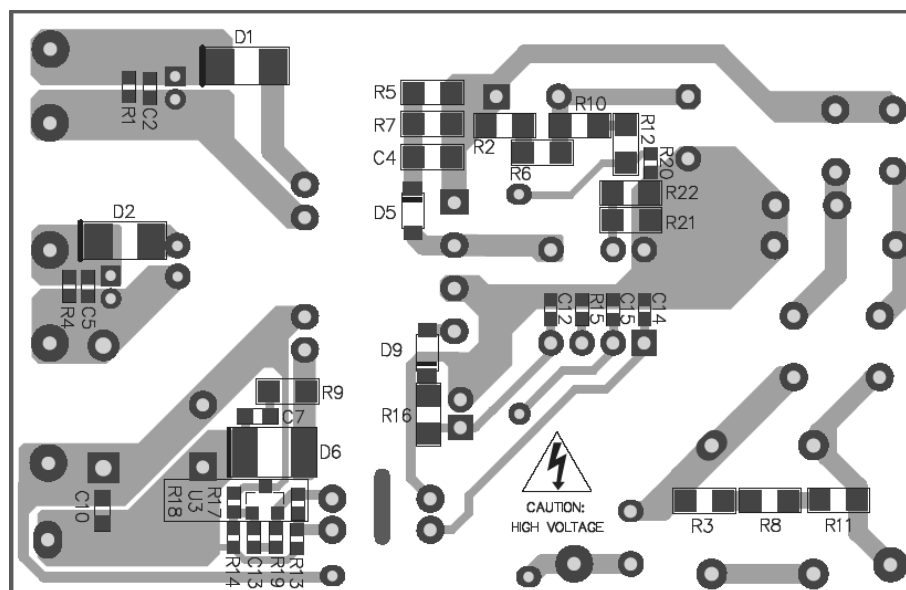
Figure 3—Bottom Layer
