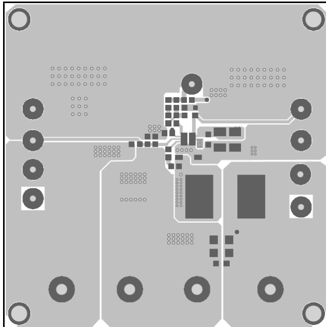
Figure 2—Top Layer
