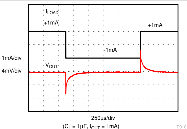
图 8-10. 负载瞬态
