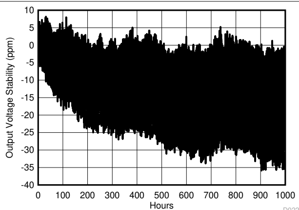
图 8-25. 长期稳定性 - 1000 小时 ( V_{REF} ) - DBV 封装
