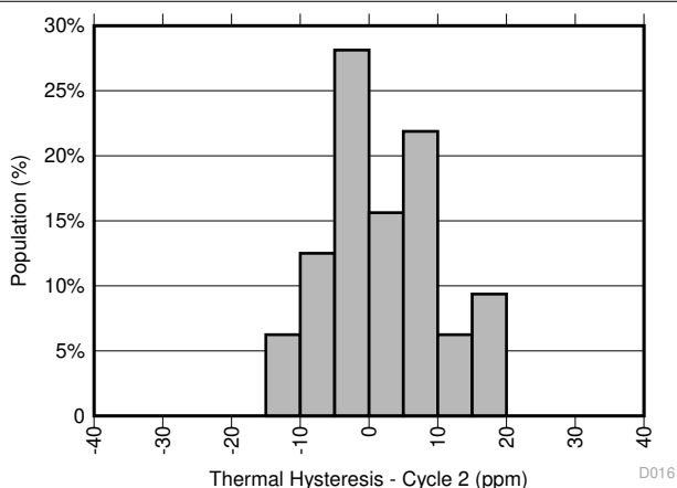
图 8-18. 热迟滞分布 (周期 2) - DBV 封装
