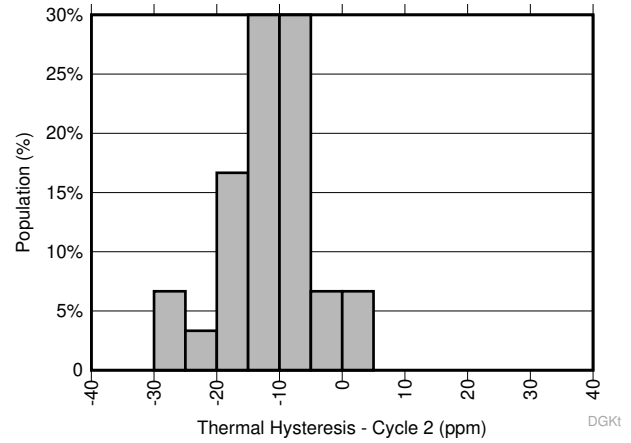
图 8-20. 热迟滞分布 ( 周期 2 ) - DGK 封装
