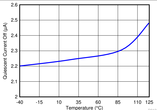
图 8-16. 关断模式下的静态电流
