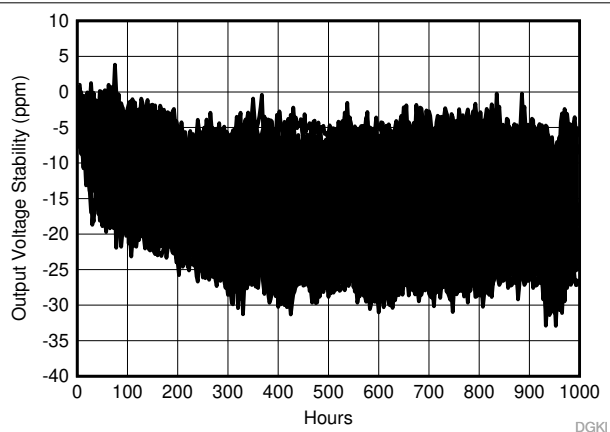
图 8-26. 长期稳定性 - 1000 小时 ( V_{REF} ) - DGK 封装
