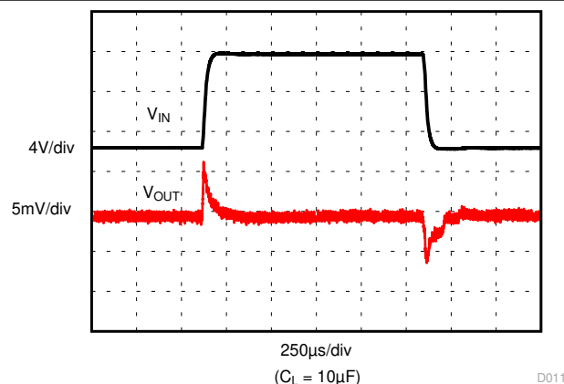
图 8-15. 线路瞬态
