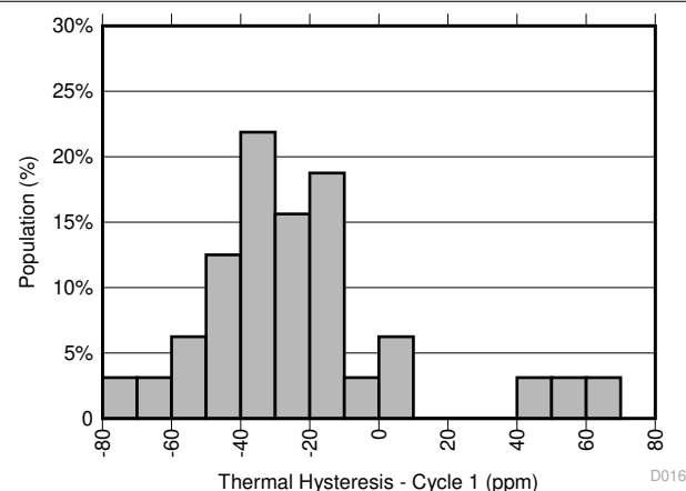
图 8-17. 热迟滞分布 (周期 1) - DBV 封装
