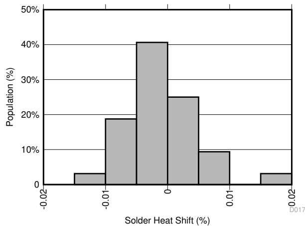
图 9-2. 焊接热漂移分布， V_{REF} (%) - DBV 封装
