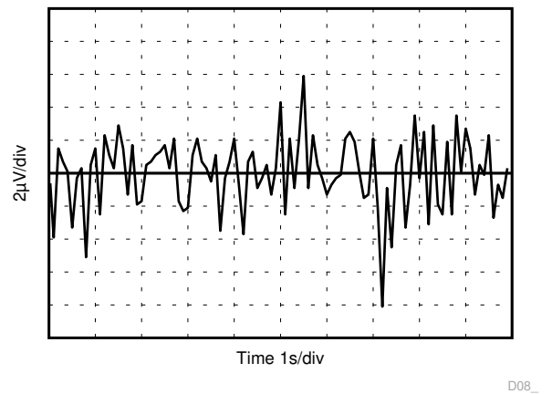
图 8-24. 0.1Hz 至 10Hz 噪声 ( V_{REF} )
