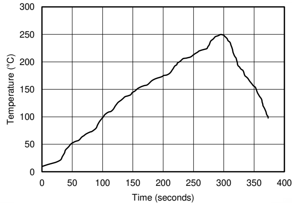
图 9-1. 回流焊曲线
