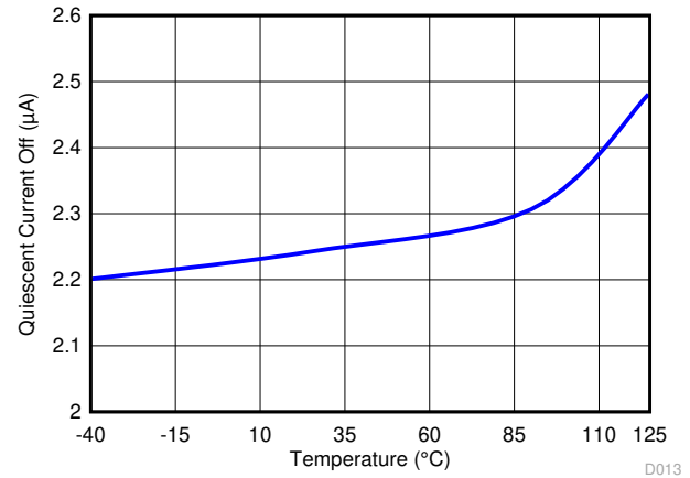
图 11-3. 关断模式下的静态电流
