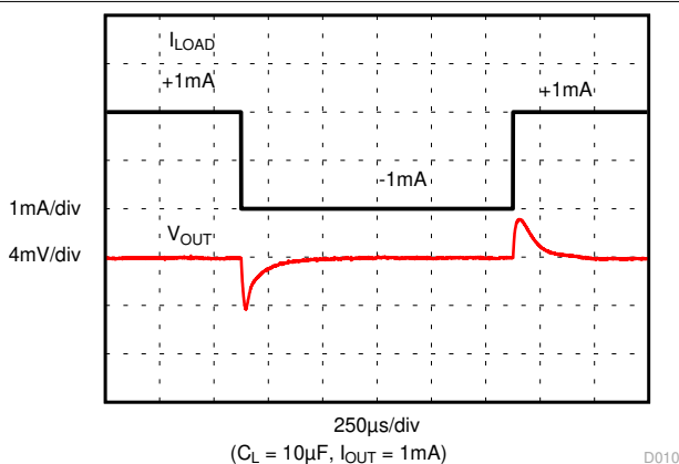
图 8-11. 负载瞬态
