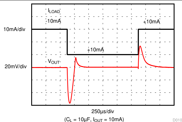
图 8-13. 负载瞬态
