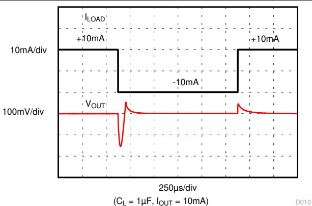
图 8-12. 负载瞬态
