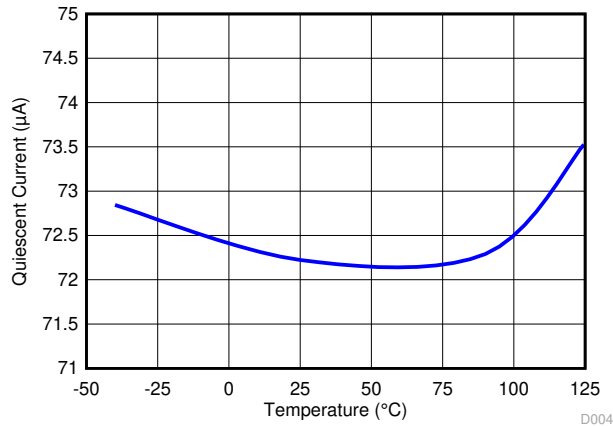
图 11-2. 静态电流与温度间的关系
