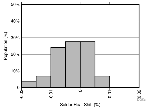
图 9-3. 焊接热漂移分布， V_{REF} (%) - DGK 封装
