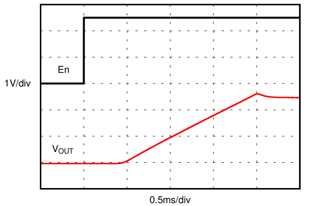
图 8-23. 导通时间 ( 启用 )
