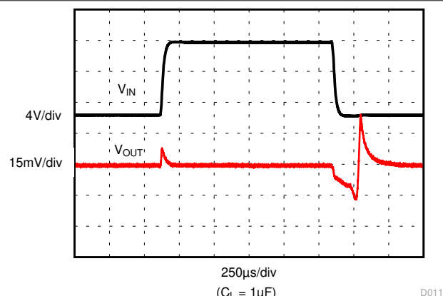
图 8-14. 线路瞬态
