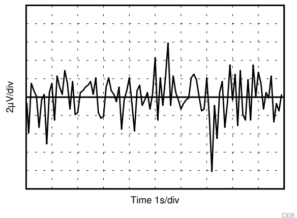
图 9-10. 0.1Hz 至 10Hz 噪声 ( V_{REF} )
