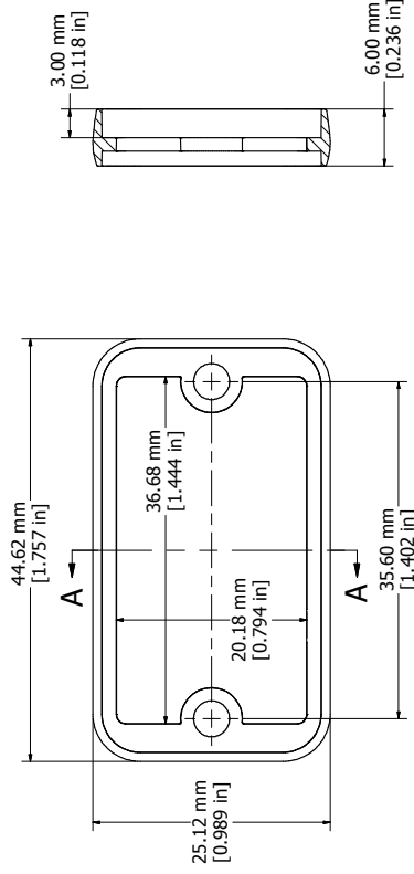
OPEN BEZEL
