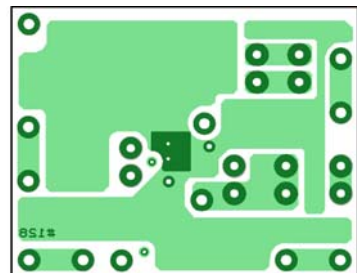
4 th Layer
