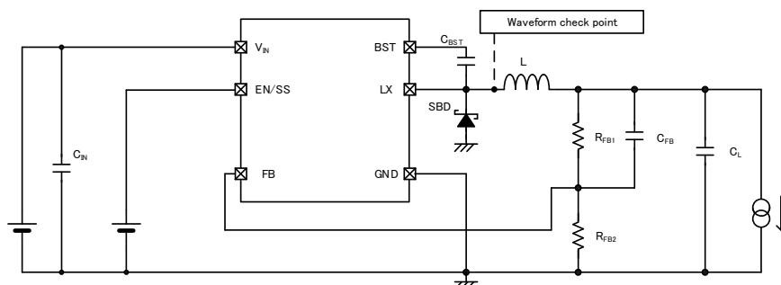
<Circuit No.①>
