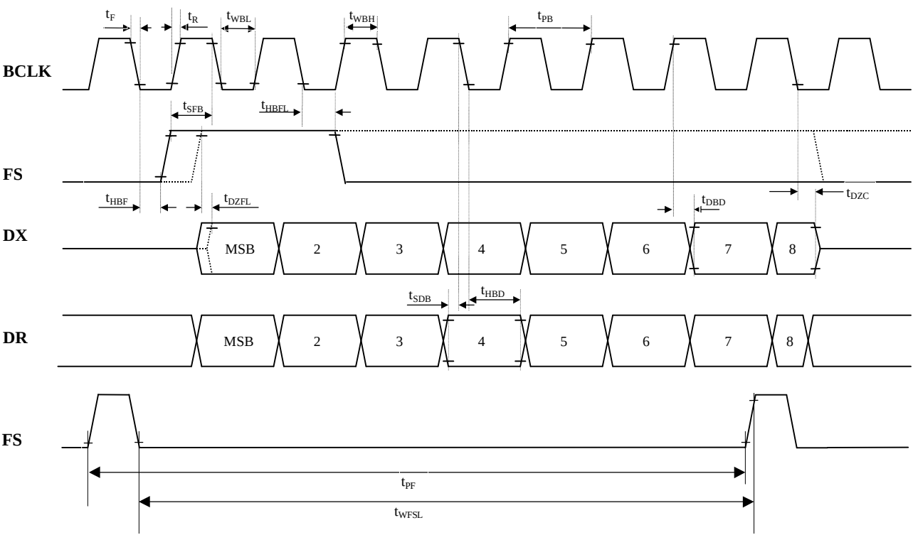
図 1 PCM Interface Timing < Long Frame >
