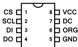
8L TSSOP
