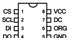
8L SOIC
