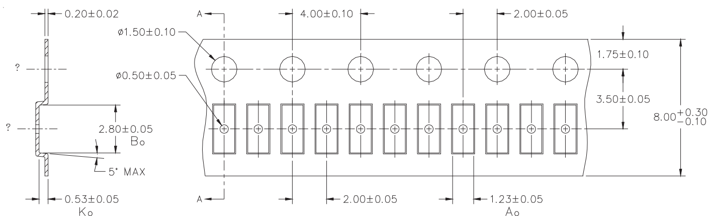
SECTION A-A
