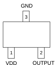
SOT23-3L
