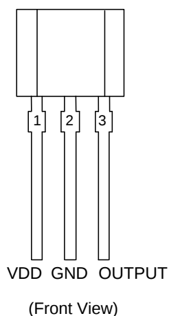
SIP-3L(TO-92S)
