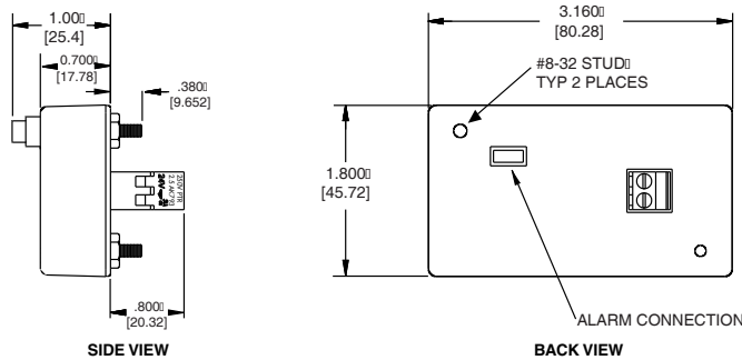
CRM3000-50-R UNIT DIMENSIONS
