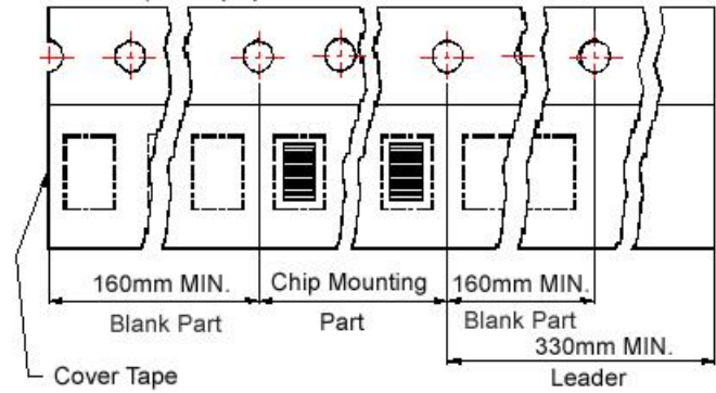
Reel Dimensions
