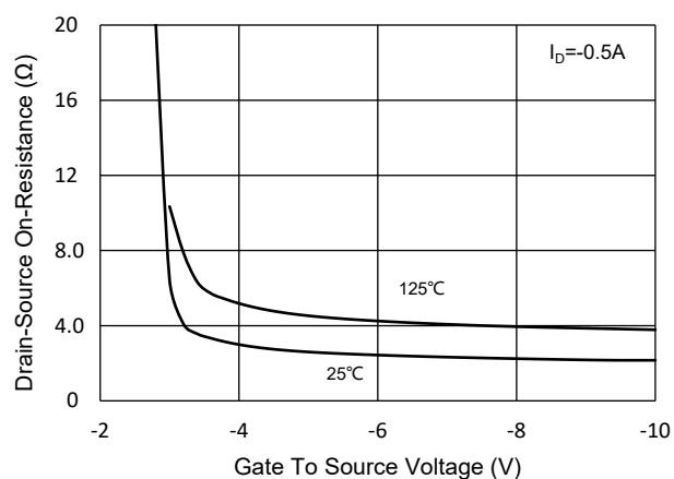
Fig.3 - R_{DS(ON)} - V_{GS}
