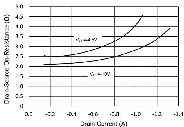
Fig.4 - R_{DS(ON)} - I_D
