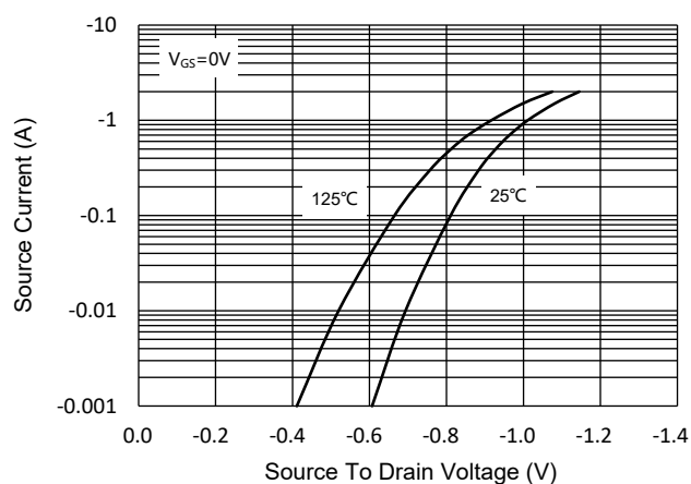
Fig.9 - I_S - V_{SD}
