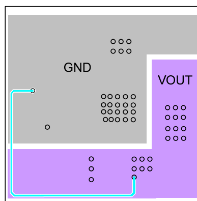
Bottom Layer
