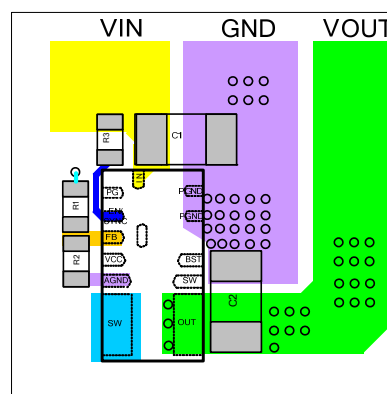
Top Layer
