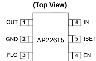
TSOT26
